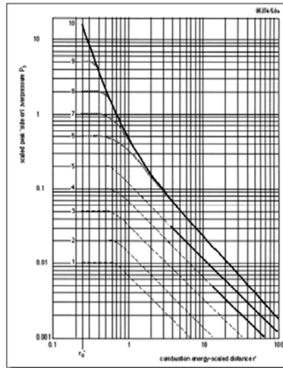
FIGURA 11 - Sobre pressão adimensional
