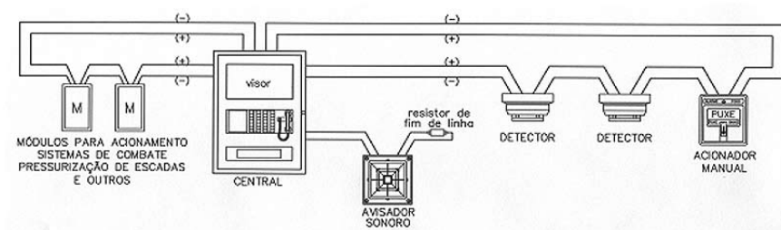
FIGURA 4: Exemplo de sistema microprocessado – circuito classe A
