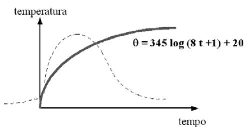
FIGURA 26 - Modelo do incêndio-padrão ISO 834
