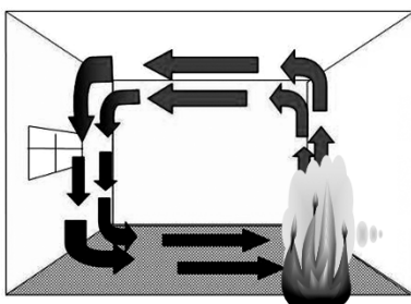
FIGURA 18 - Convecção decorrente de um incêndio
