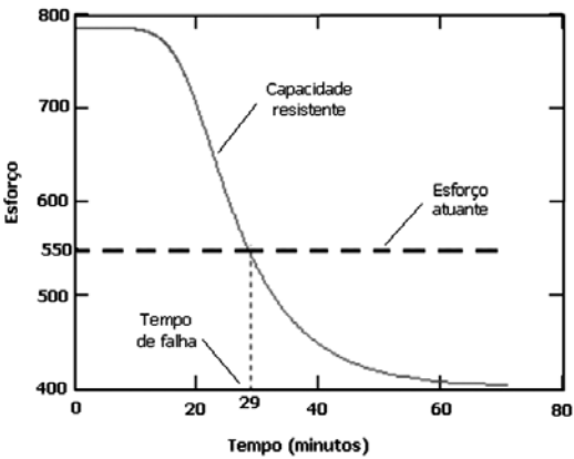
FIGURA 13 - Redução da resistência de uma seção de um elemento estrutural quando ( S_{\text{incêndio}} = R_{\text{incêndio}} )
