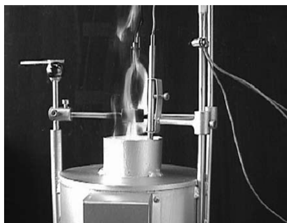
FIGURA 3: Equipamento de ensaio de não-combustibilidade
