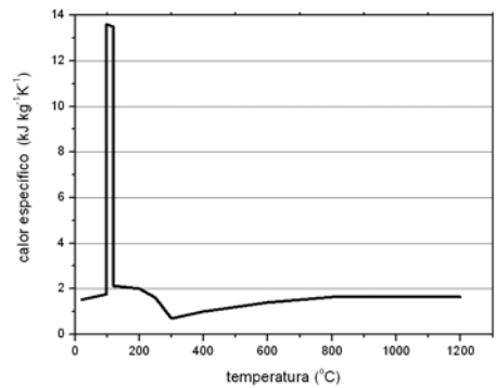
FIGURA 16 - Calor específico da madeira e camada carbonizada
