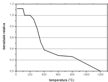
FIGURA 17 - Densidade para U inicial de 12%
