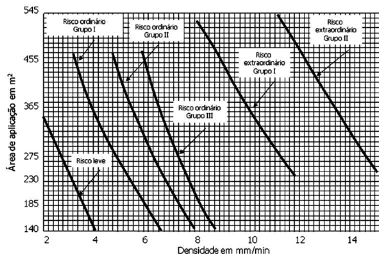
FIGURA 10 - Área de aplicação e densidade em função da classe de risco de ocupação (NBR 10897 (1990))
