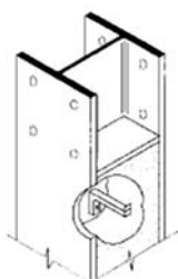
FIGURA 41 - Pilares mistos de aço e concreto solidarizados por intermédio de conectores de cisalhamento, fornecem proteção de 60 minutos
