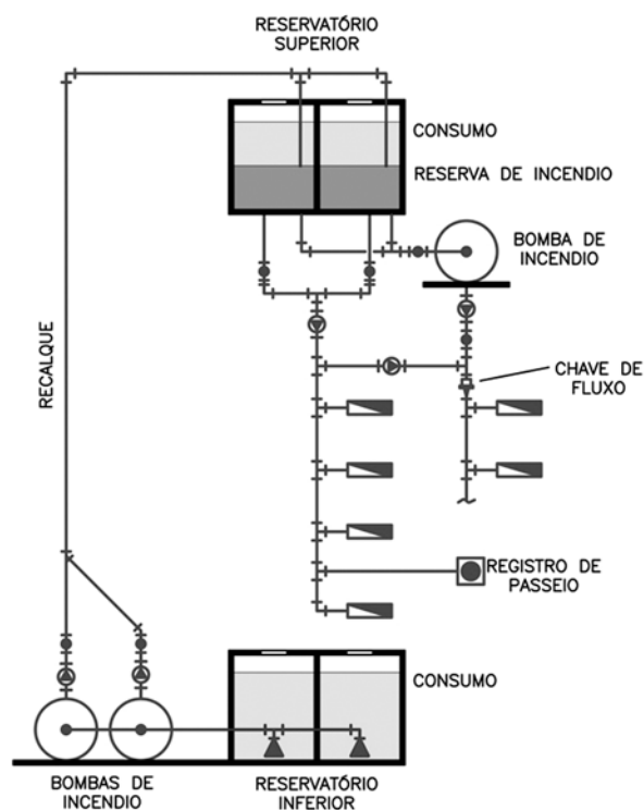
FIGURA 3 - Sistema de hidrantes por gravidade e bomba de incêndio (GONÇALVES (1993))
