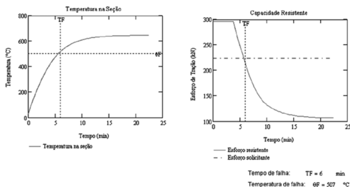
FIGURA 17 - Temperatura e capacidade resistente da seção versus tempo para o caso 1 submetido a uma energia térmica radiada de 28,4 kW/m²
