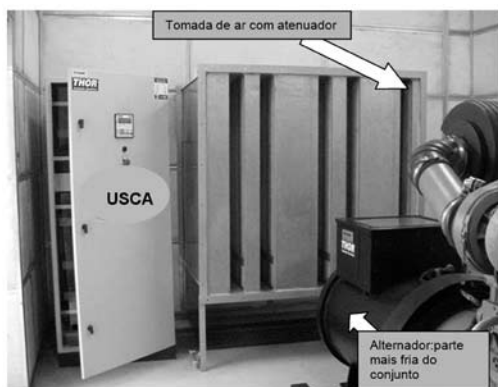
FIGURA 1: Outros detalhes do leiaute da sala do gerador – tomada de ar
