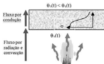
FIGURA 20 - Fluxo de calor através de um elemento de compartimentação
