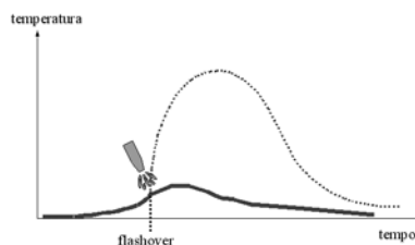
FIGURA 23 - Curva temperatura-tempo de um incêndio afetado pela presença de chuveiros automáticos
