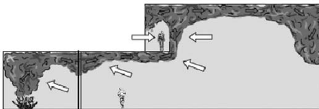
FIGURA D As setas representam o movimento previsto da fumaça, enquanto as setas brancas mostram a direção do movimento do ar fresco sem a ventilação da fumaça
