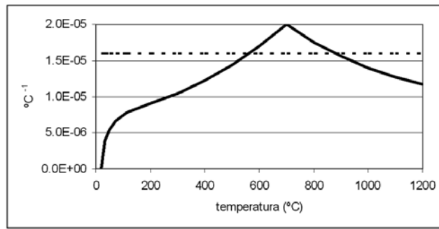
FIGURA 11 - Coeficiente de dilatação térmica do concreto silicoso
