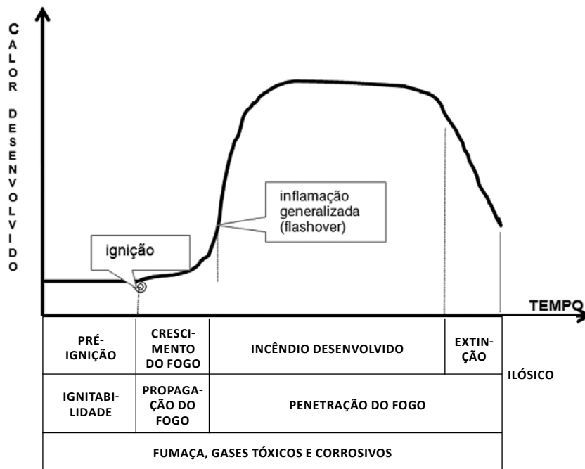
FIGURA 7: Curva de evolução do incêndio celulósico
